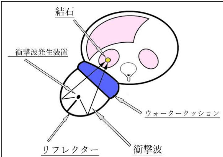
図1：対外衝撃波結石破砕術
