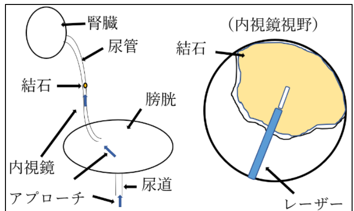
図2：経尿道的結石破砕術
